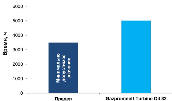
Термоокислительная стабильность*
