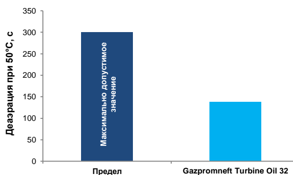
Деаэрационные свойства**
