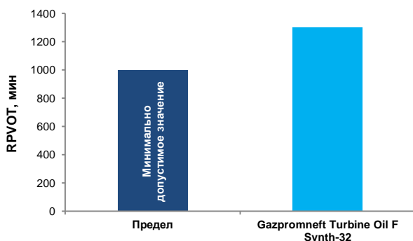
Термоокислительная стабильность*
